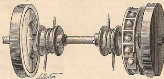
FIG. 1. — Dessin descriptif, Poulie Mtrice de la Pédale Magique Bâcle . Pied moteur avec bobines d'encliquetage à boules libres. Modèle perfectionné.
